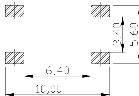
PCB. 焊接图
